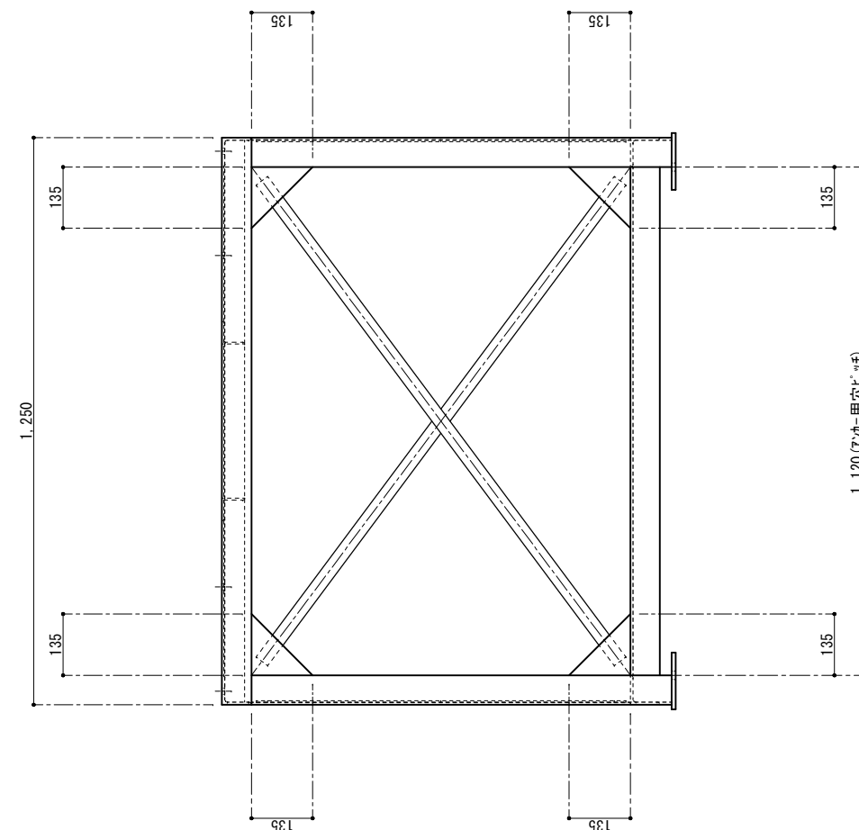
⑤ アンカープレート詳細
