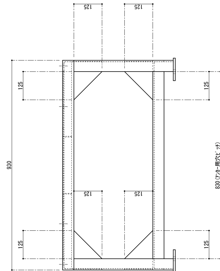
⑤ アンカープレート詳細
